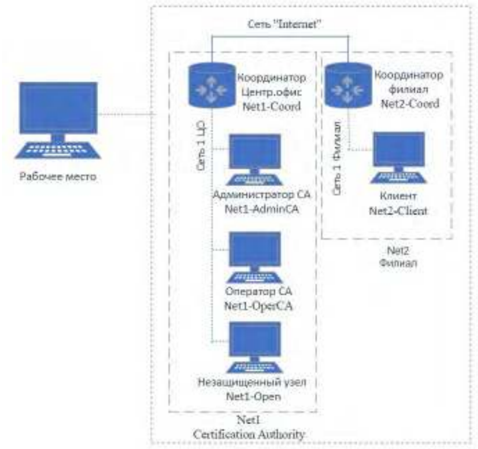
Рисунок 1 Схема защищенной сети
